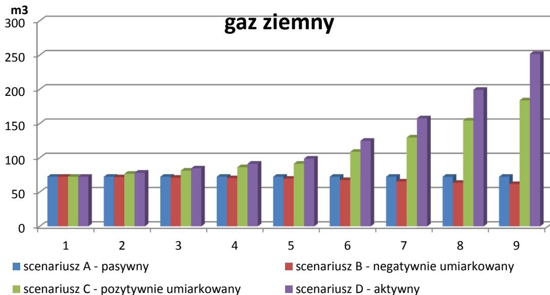
Rys. 31 Scenariusze zużycia gazu ziemnego do roku 2030
