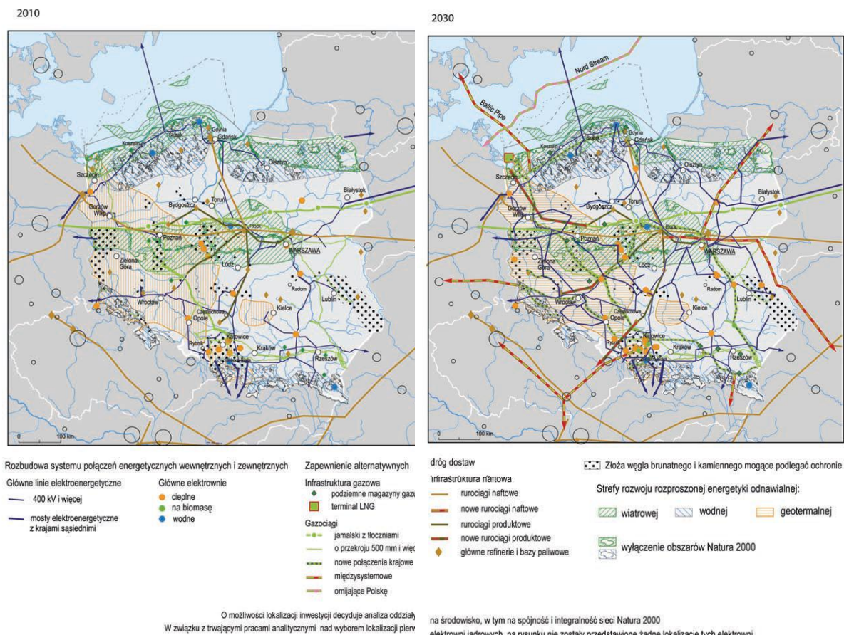
Rys. 21 System energetyczny i kierunki rozwoju energetyki odnawialnej w 2010 i 2030 roku
