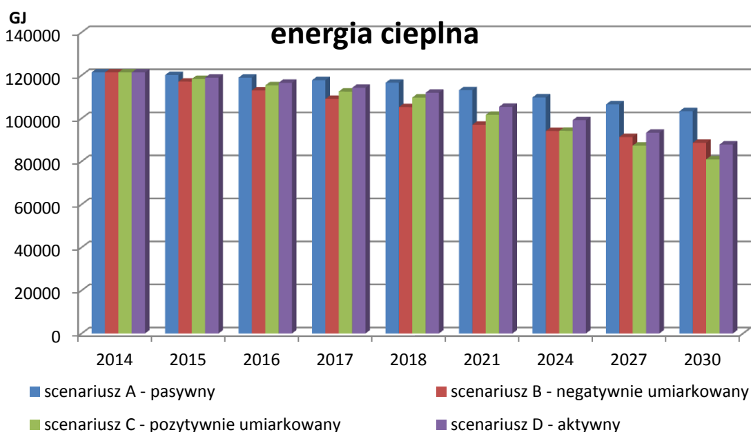
Rys. 29 Scenariusze zużycia energii cieplnej do roku 2030
