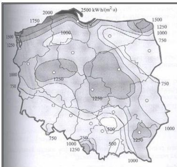
Rys. 19 Teoretyczna gęstość mocy wiatru (wyrażona w kWh/(m 2 *a)) na wysokości 30 m n.p.g.
