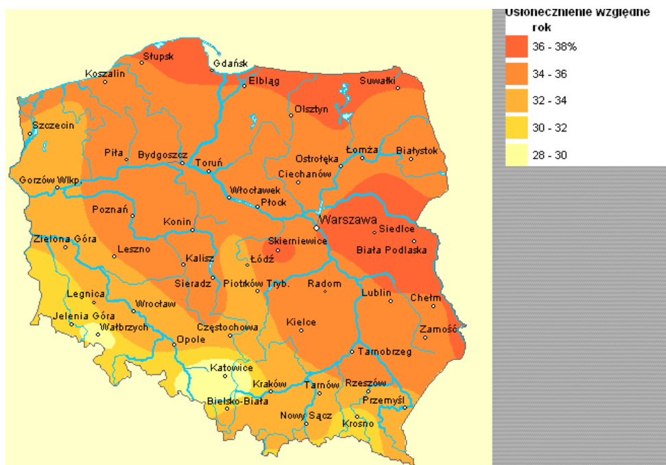
Rys. 23 Uśonecznienie względne Polski
