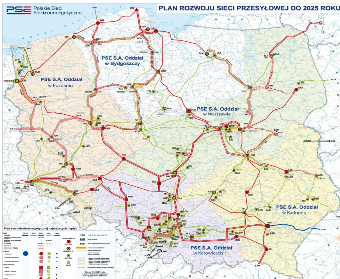
Rys. 14 Schemat Krajowego Systemu Przesyłowego (KSE)
