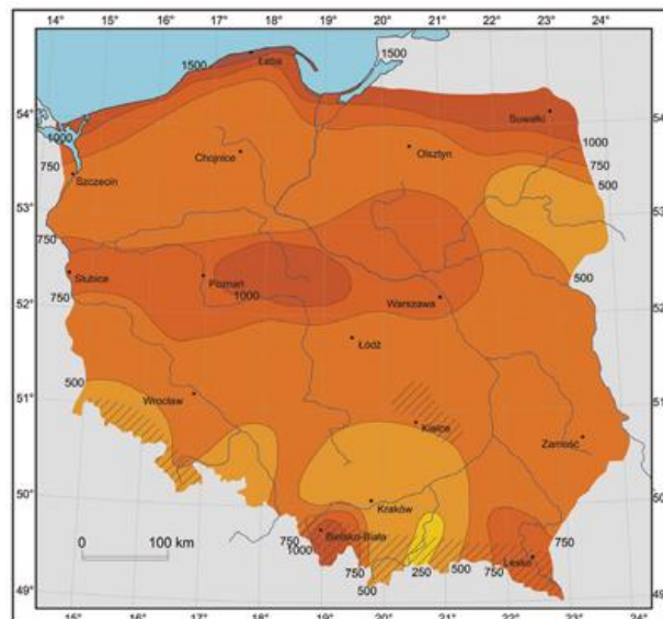
Rys. 20 Teoretyczna gęstość mocy wiatru (wyrażona w kWh/(m 2 *a)) na wysokości 10 m n.p.g. w terenie otwartym o niskiej szorstkości.
