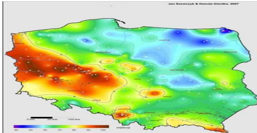
Rys. 27 Mapa strumienia ciepłego Polski
