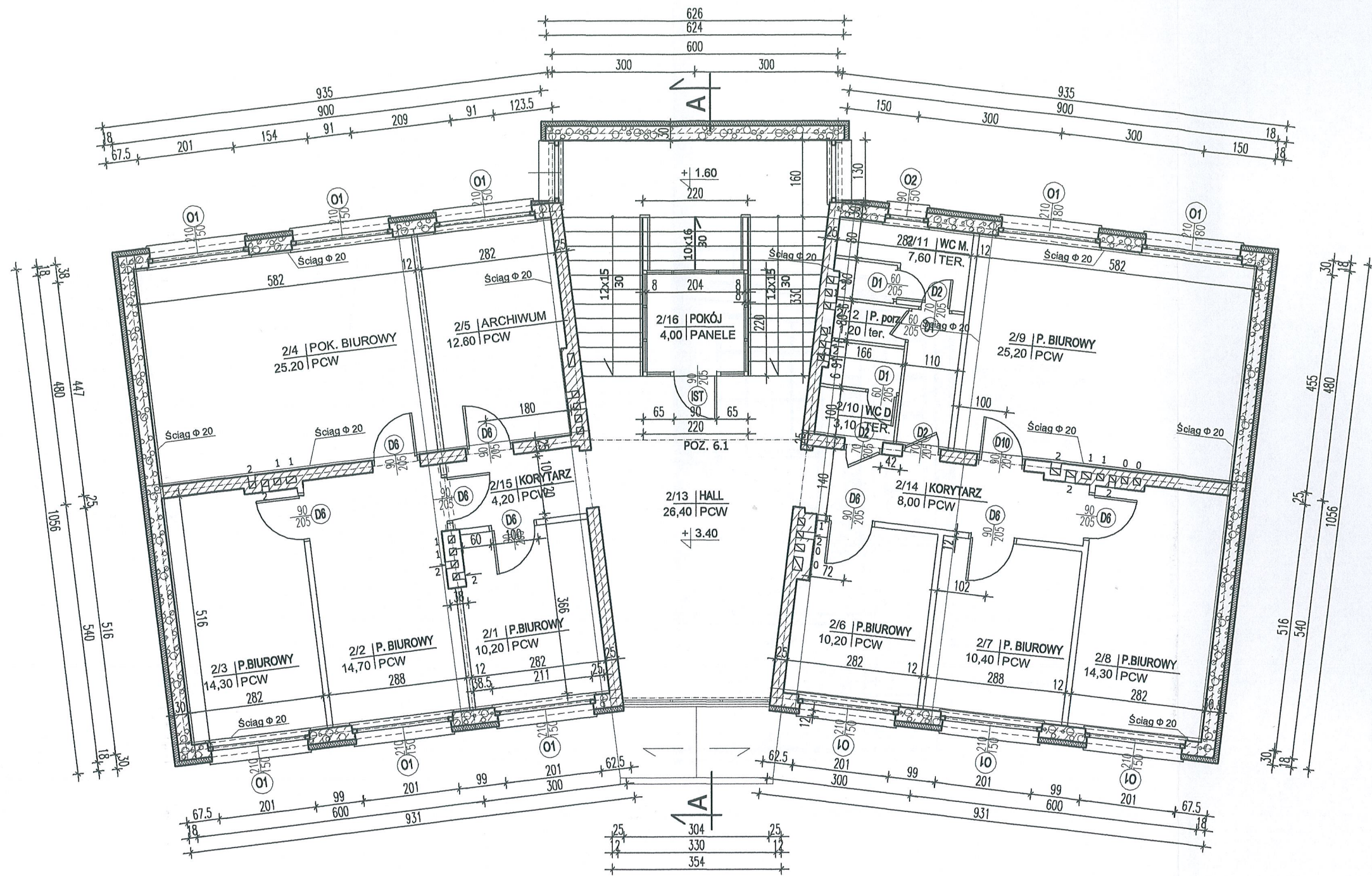
RZUT PIĘTRA 1:100
